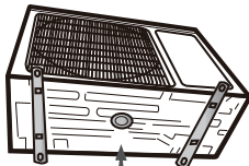
foro di scarico base unità esterna giunto di scarico condensa tubo di scarico condensa
